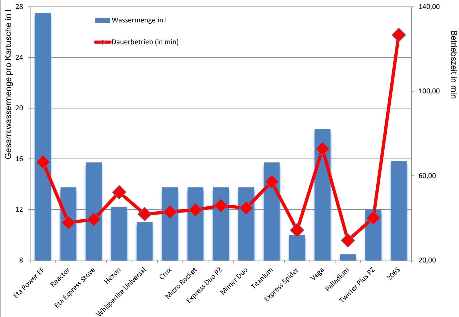
Vergleich: Wassermenge (Volumen in l) vs. Dauerbetrieb des Kochers (Zeit in min)
