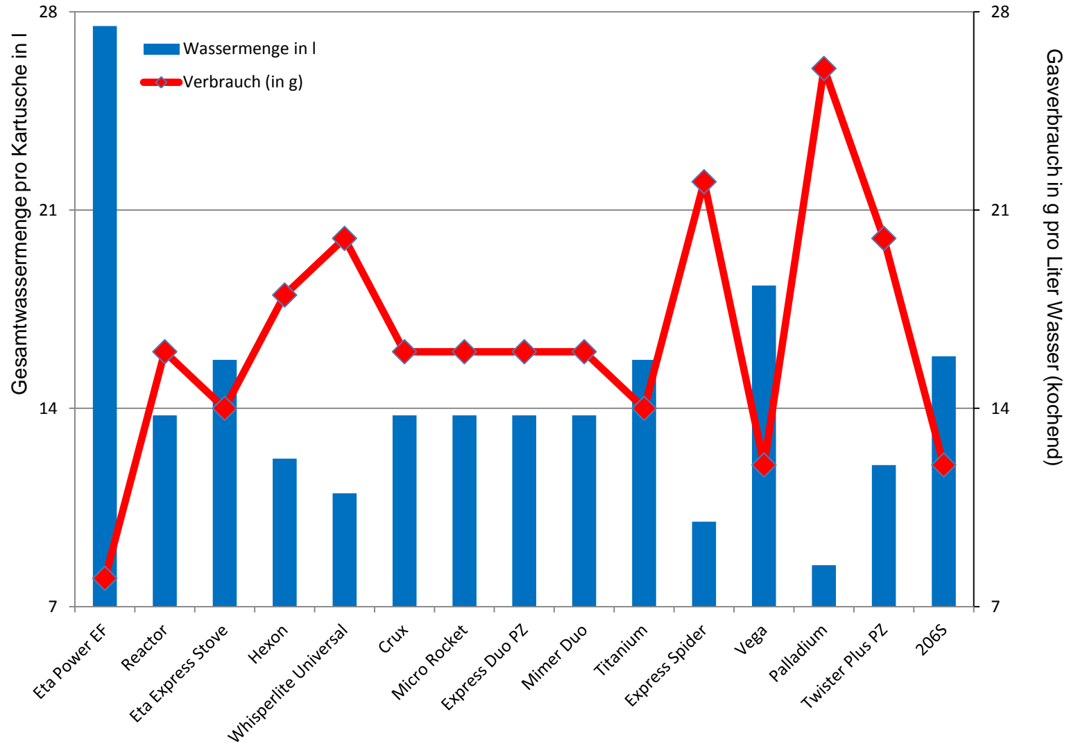
Vergleich: Wassermenge (Volumen in l) vs. Gasverbrauch pro 1l Wasser kochend (Menge in g)
